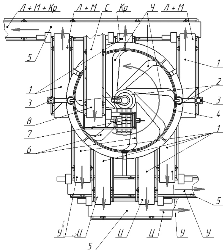
1 – транспортер; 2 – привод карусели; 3 – привод подъемника; 4 – стенка бункера; 5 – конвейер; 6 – пневмоканал; 7 – пробник; 8 – транспортер зернового вороха.
