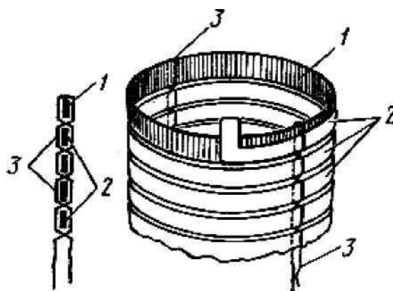
Рис.3. Пример закрепления витков и уравнивательного клиновидного поиска:
