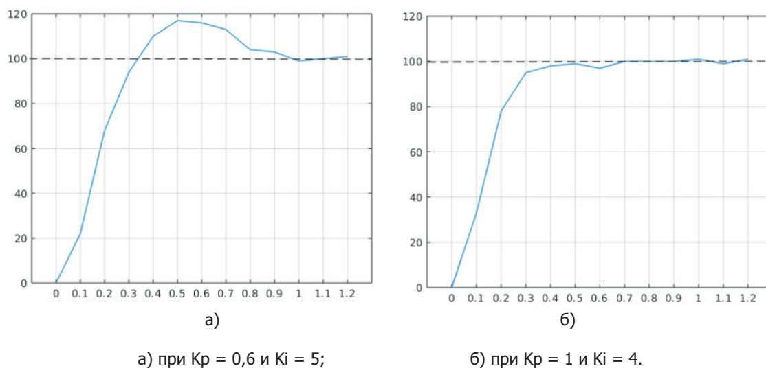
Рисунок 9 – Поведение двигателя
