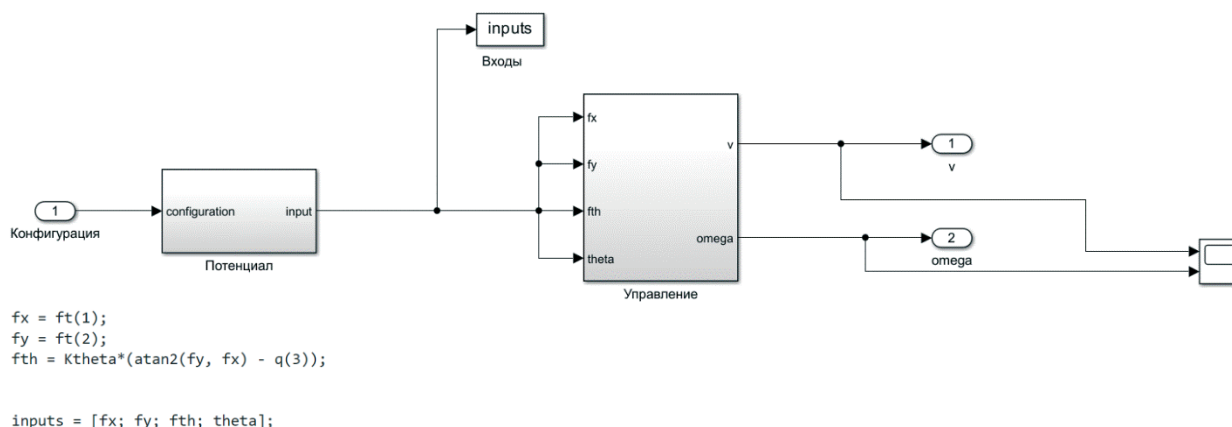
Рисунок 3 – Регулятор искусственного потенциального поля
