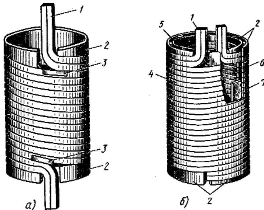
Рис.1. Цилиндрические обмотки:
