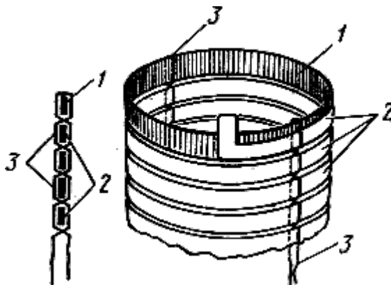
Рис.3. Пример закрепления витков и уравнительного клиновидного поиска:
