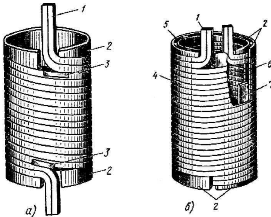
Рис.1. Цилиндрические обмотки:
