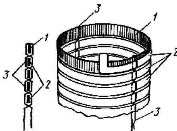
Рис.3. Пример закрепления витков и уравнивающего клиновидного поиска:
