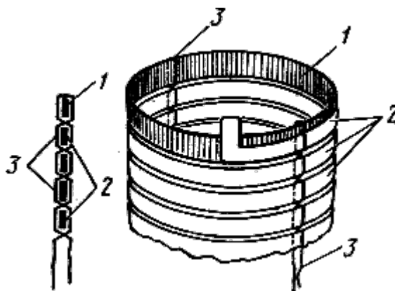
Рис.3. Пример закрепления витков и уравнивательного клиновидного пояска:
