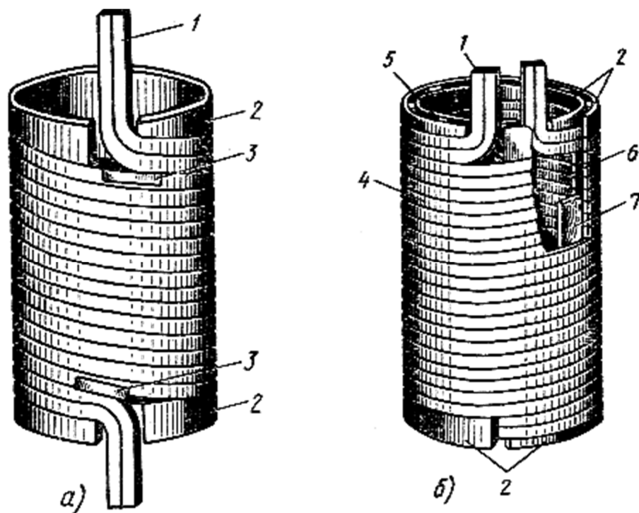
Рис.1. Цилиндрические обмотки:
